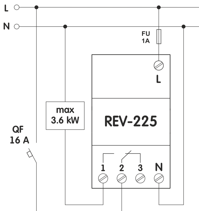
Рисунок 2 – Схема підключення REV-225
