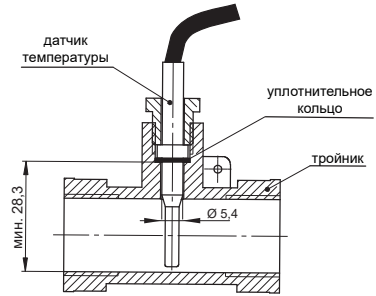
Рис. 2 Установка датчика в шаровом клапане
