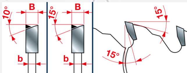
Змінний зуб 10°
