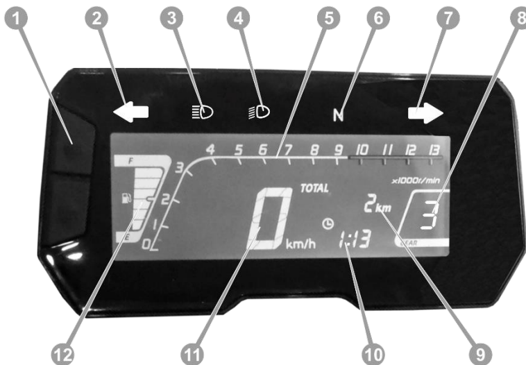
Рисунок 3.2 – Панель приладів*
