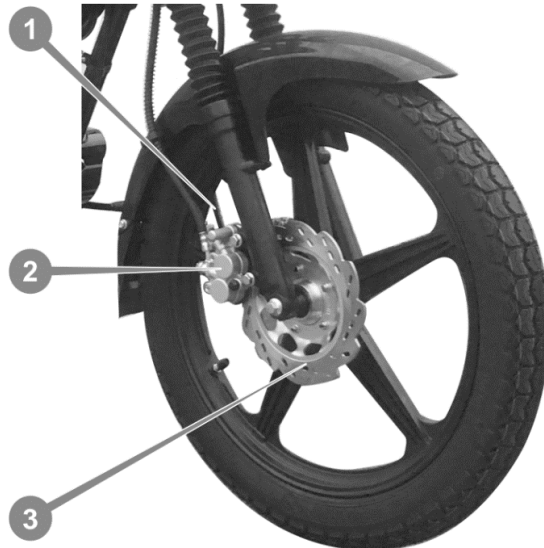
Рисунок 17. Переднє гальмо
