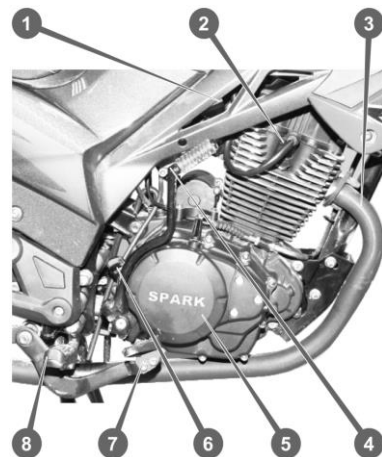
Рисунок 3.6. Силовий агрегат, вид справа
