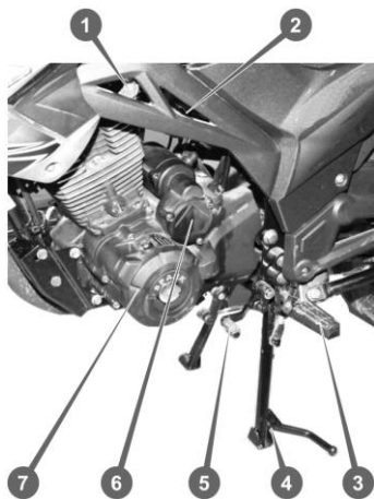
Рисунок 3.5. Силовий агрегат, вид зліва
