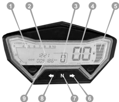
Рисунок 3.3. Панель з дисплеєм
