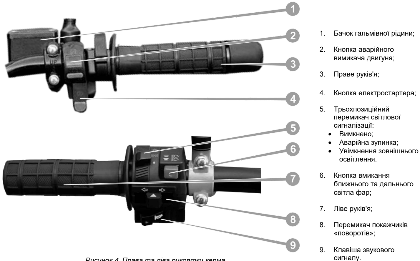
Рисунок 4. Права та ліва рукоятки керма
