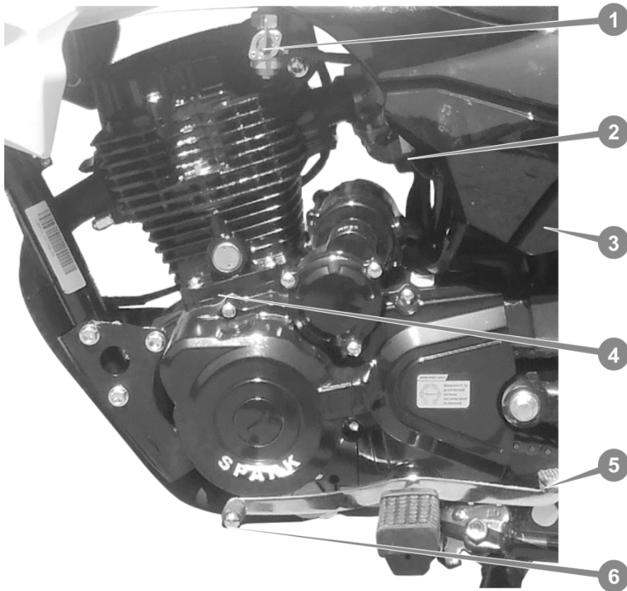
Рисунок 5. Вид двигуна ліворуч
