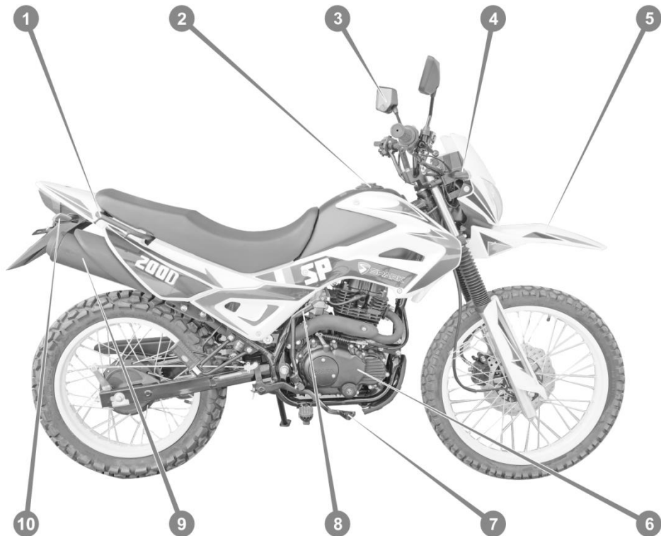
Рисунок 2. Мотоцикл, вид праворуч
