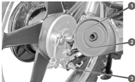
Рисунок 18. Заднє гальмо
