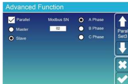
Підлеглий інвертор
