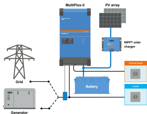
Паралельне використання в мережі з MPPT контролером сонячного заряду
