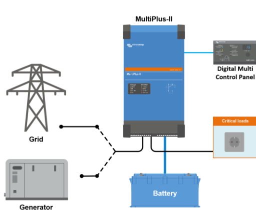
Стандартне застосування в морі, мобільне або автономне застосування
