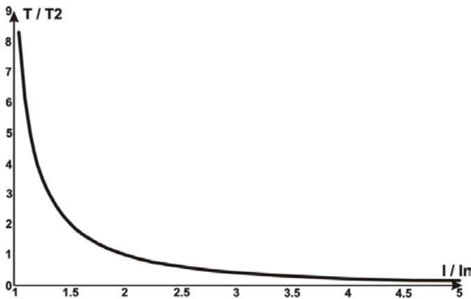
Рисунок 6 – Токо-временная характеристика
