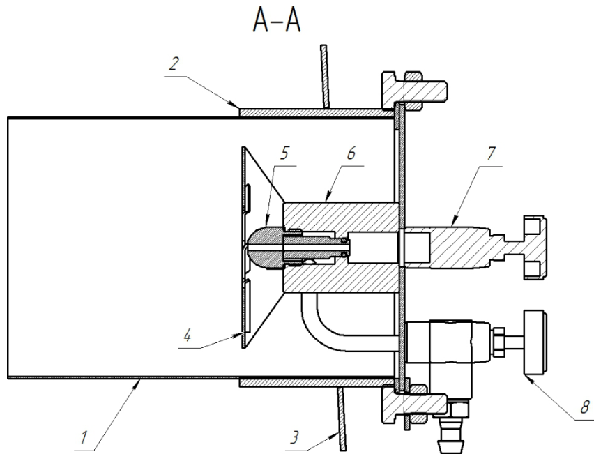
1. Допалювач 2. Жарова труба 3. Монтажний фланець 4. Завихрювач 5. Форсунка 6. Адаптер 7. Повітряний вентиль 8. Паливний вентиль Малюнок №1
