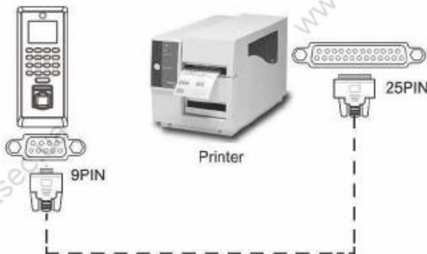
[Диаграмма подключения]
