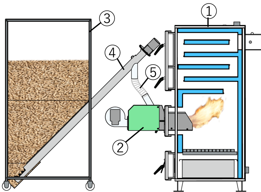
Мал. 8 – Схема установки пальника і пристрою подачі
