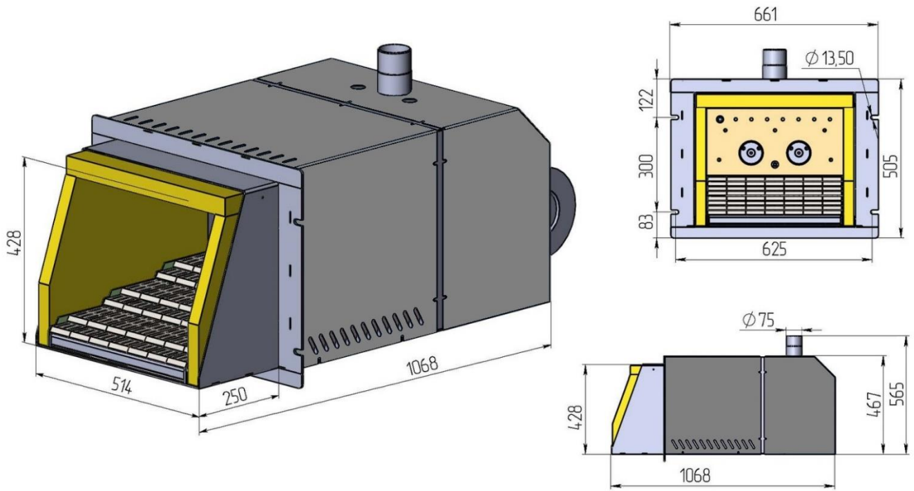
Мал. 7 – Габаритні розміри пальника «METALEX» 500 кВт
