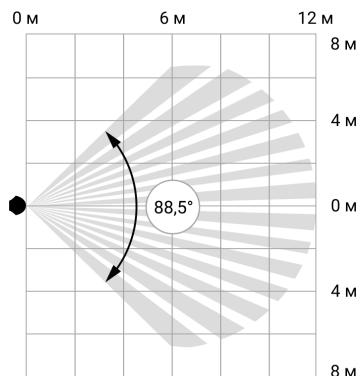
Горизонтальний кут огляду датчика
