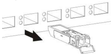
Рисунок 14 Пример удаления трансивера
