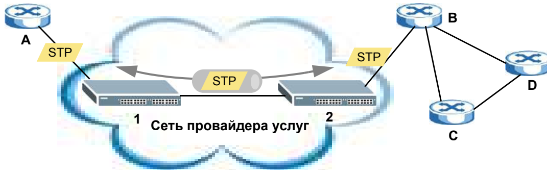
Рисунок 159 Пример сети с использованием L2PT
