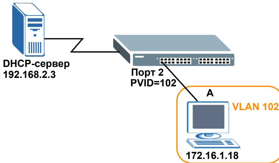
Рисунок 32 Пошаговые указания: Сценарий ретрансляции DHCP
