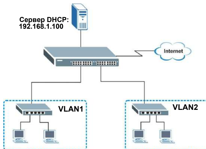
Рисунок 202 Пример сети с глобальной ретрансляцией DHCP
