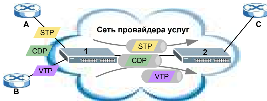
Рисунок 158 Сетевой сценарий туннелирования протоколов уровня 2
