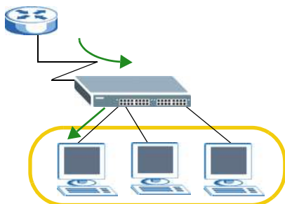
Рисунок 76 Многоадресная рассылка на основе статических адресов на два и более портов
