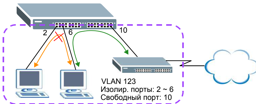
Рисунок 171 Пример частной сети VLAN
