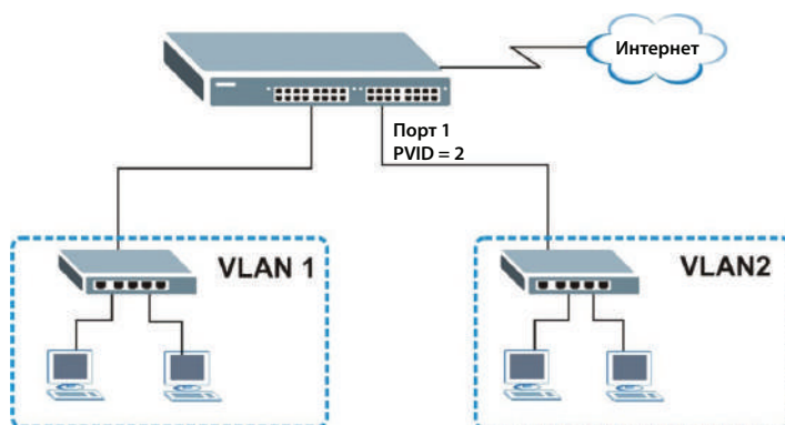
Рисунок 23 Пример первичной настройки сети: идентификатор виртуальной локальной сети для порта
