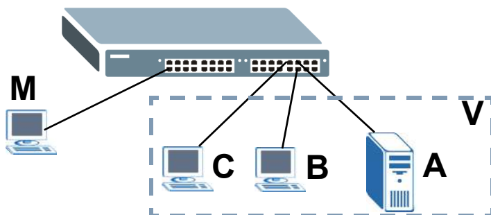
Рисунок 25 Пошаговые указания: Обзор пошаговых указаний по работе с функцией отслеживания DHCP
