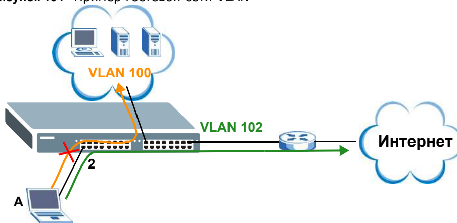
Рисунок 104 Пример гостевой сети VLAN
