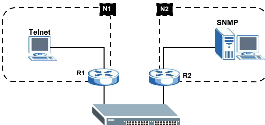
Рисунок 190 Обзор статических маршрутов
