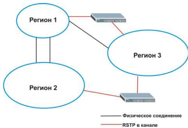
Рисунок 92 Пример сети с использованием MSTP и традиционного протокола RSTP
