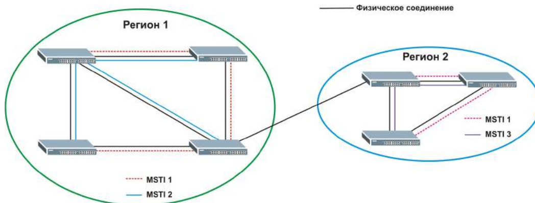
Рисунок 91 Экземпляры MSTI в различных регионах
