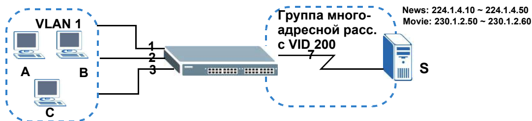
Рисунок 129 Пример настройки MVR
