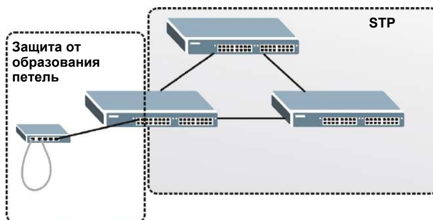
Рисунок 153 Защита от образования петель и STP
