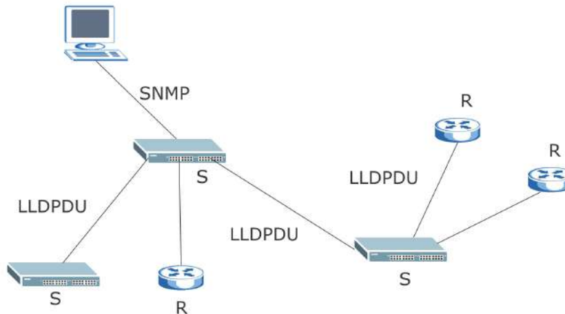
Рисунок 174 Обзор протокола LLDP
