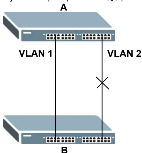
Рисунок 89 Пример сети с поддержкой STP/RSTP
