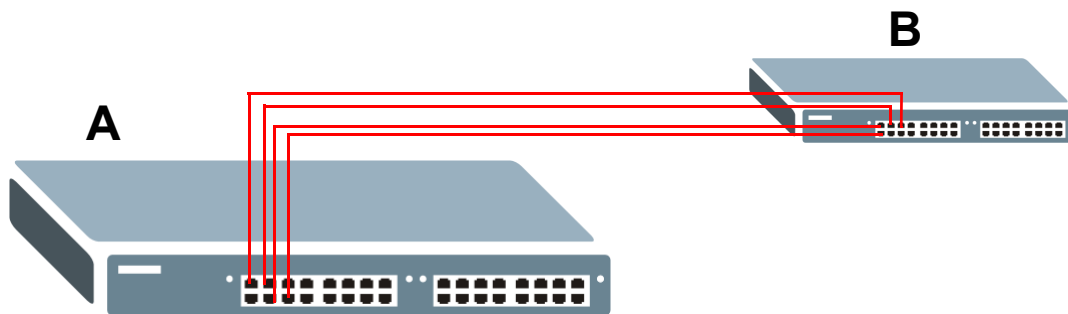
Рисунок 99 Пример группирования портов – физические подключения
