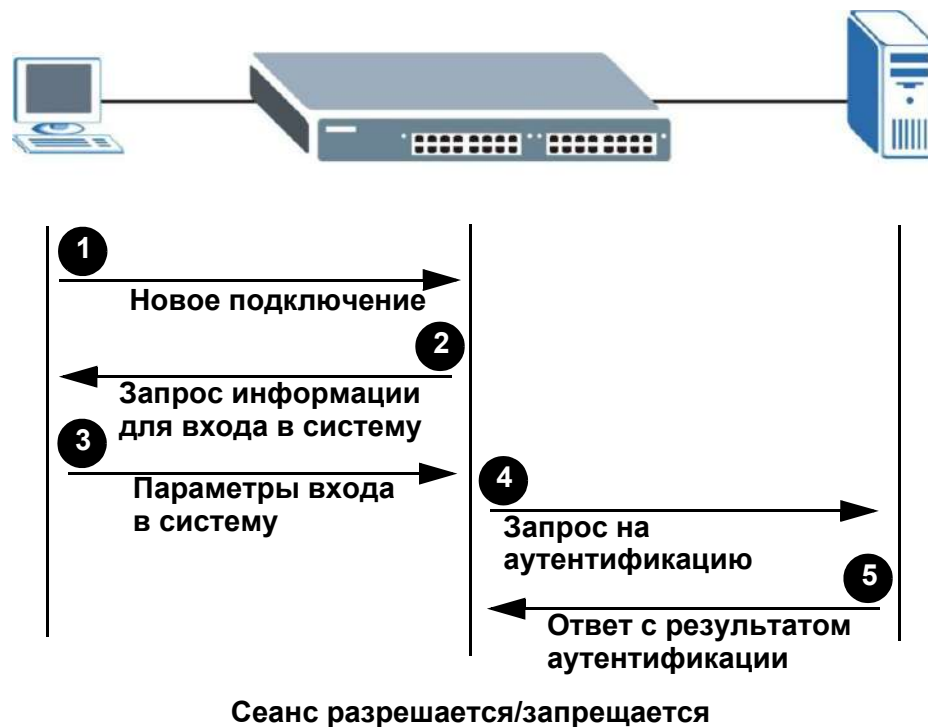
Рисунок 101 Процесс аутентификации на основе IEEE 802.1x
