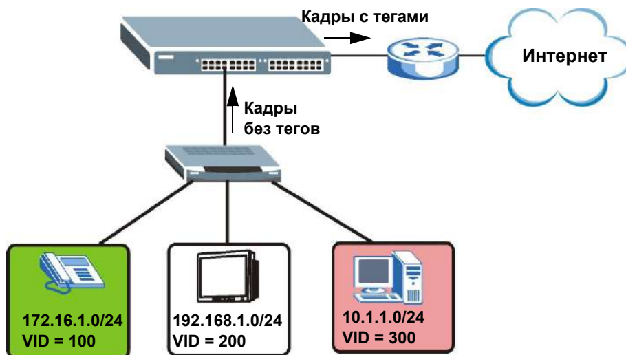
Рисунок 64 Пример использования VLAN на основе подсетей
