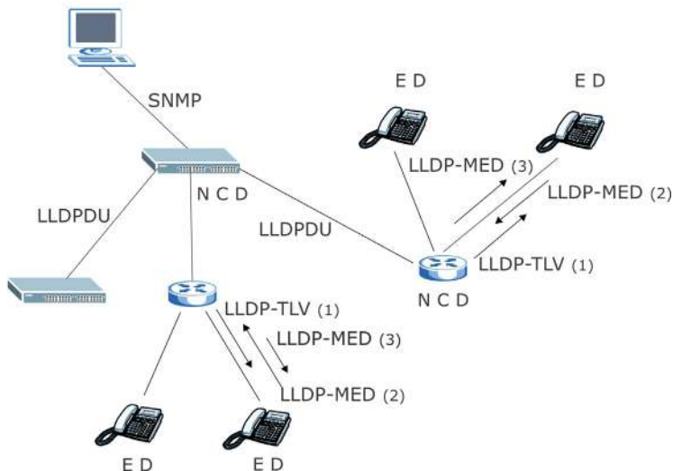
Рисунок 175 Обзор LLDP-MED
