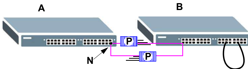
Рисунок 155 Защита от образования петель – пробный пакет
