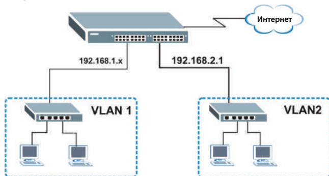
Рисунок 24 Пример первичной настройки: IP-адрес управления
