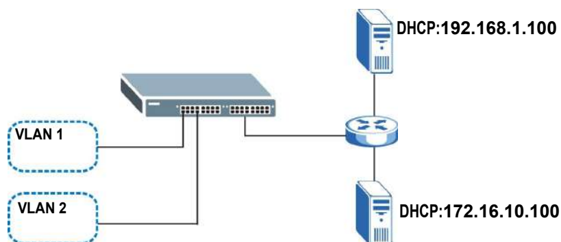
Рисунок 206 Ретрансляция DHCP для двух VLAN
