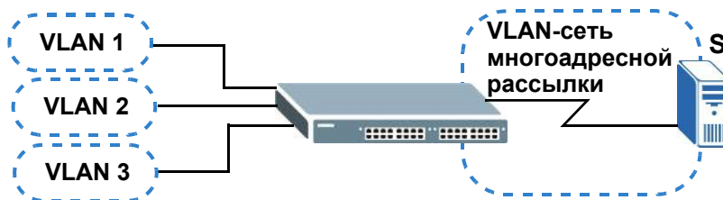
Рисунок 114 Пример сети с поддержкой MVR
