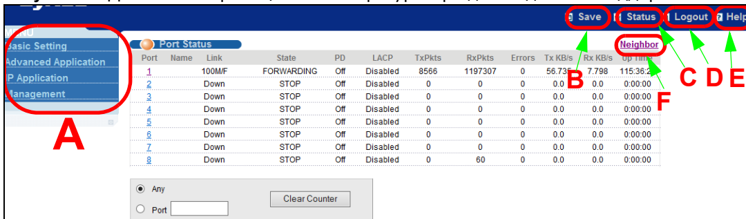
Рисунок 19 Домашняя страница Web-конфигуратора для моделей с поддержкой PoE (Status)
