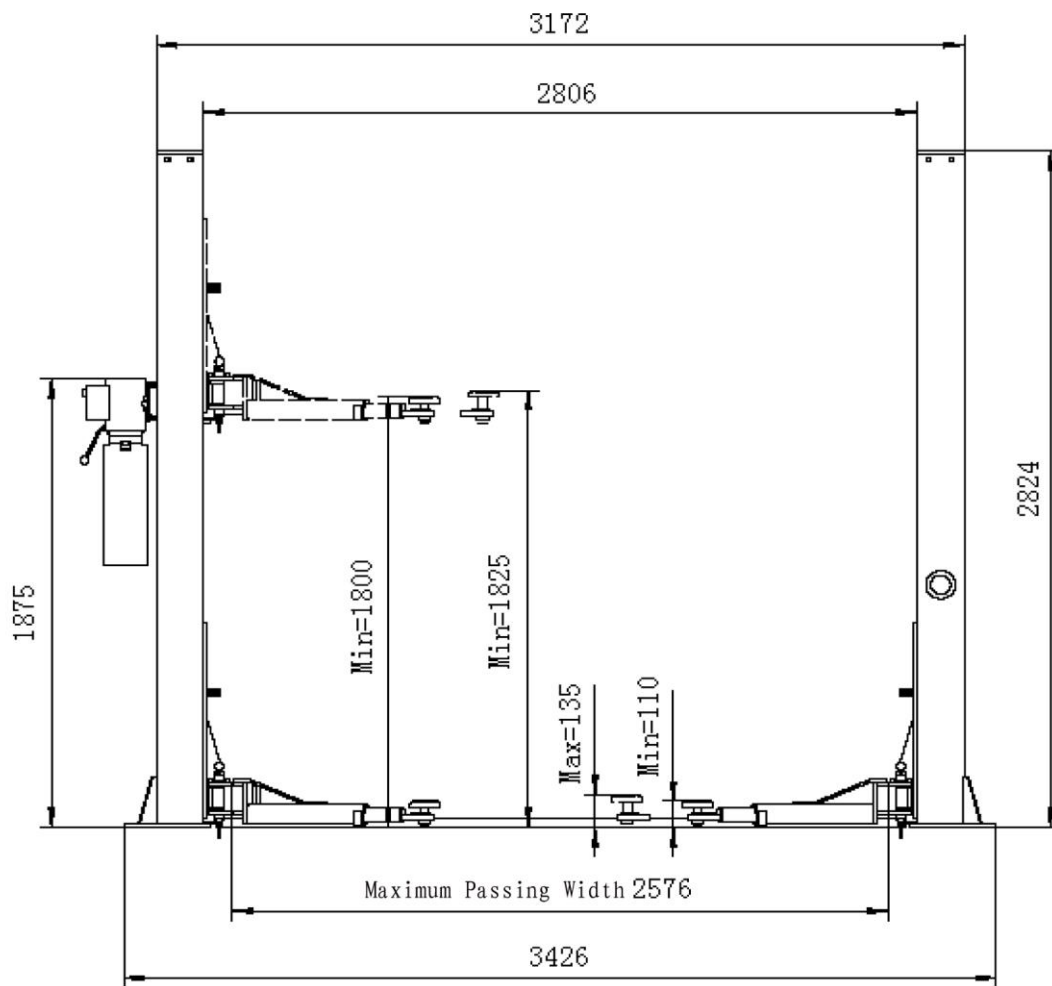
Чертеж of PL-4.0-2B:
