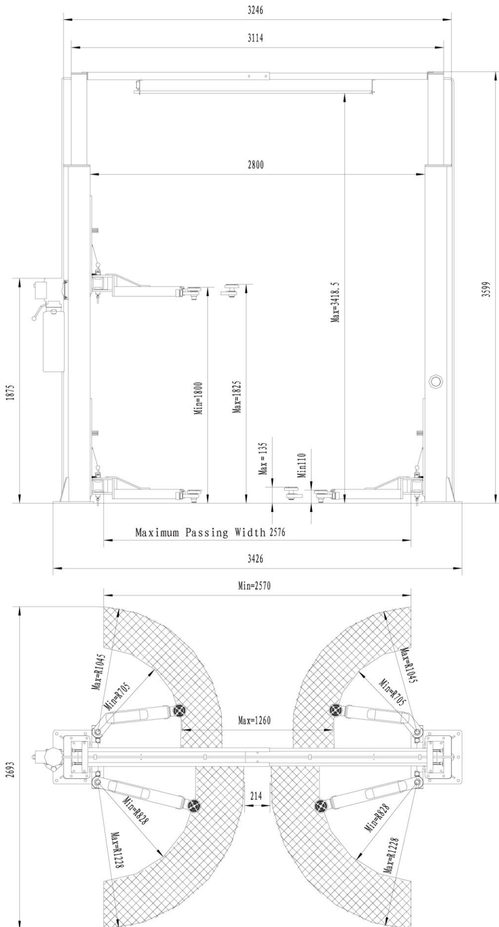
Чертеж of PL-3.8-2A:
