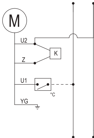
COLLEGAMENTO ELETTRICO 230V MON. AC 230V AC 1PH. ELECTRIC WIRING
