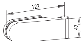
20.300.0500 петля осьова з ковпачком
