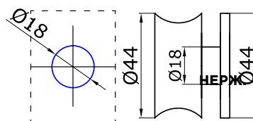
MG-1F 19 ролик під трубу 19 мм
