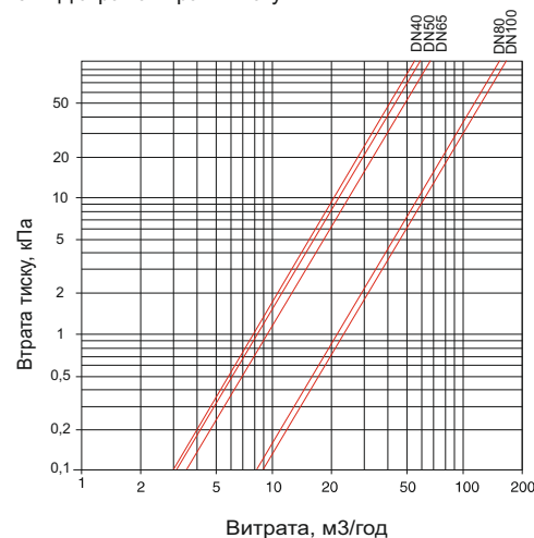
3.2. Діаграма втрати тиску
