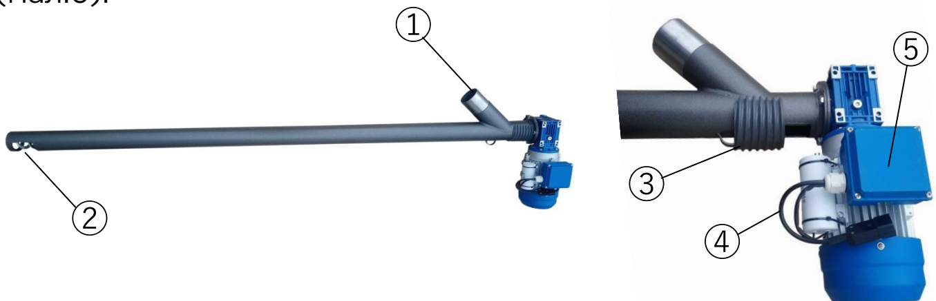
Мал.6 – Шнек подачі пелет
