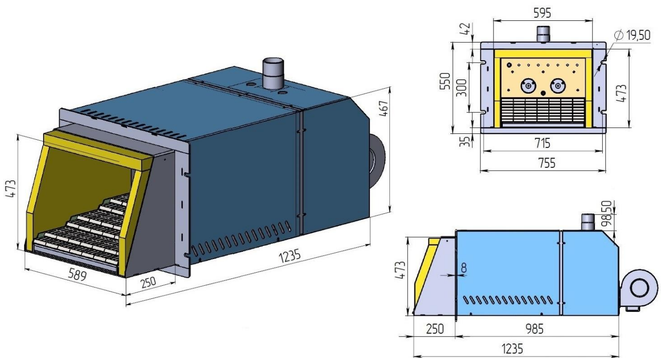
Мал. 4 - Габаритні розміри пального «METALEX» 1000 кВт
