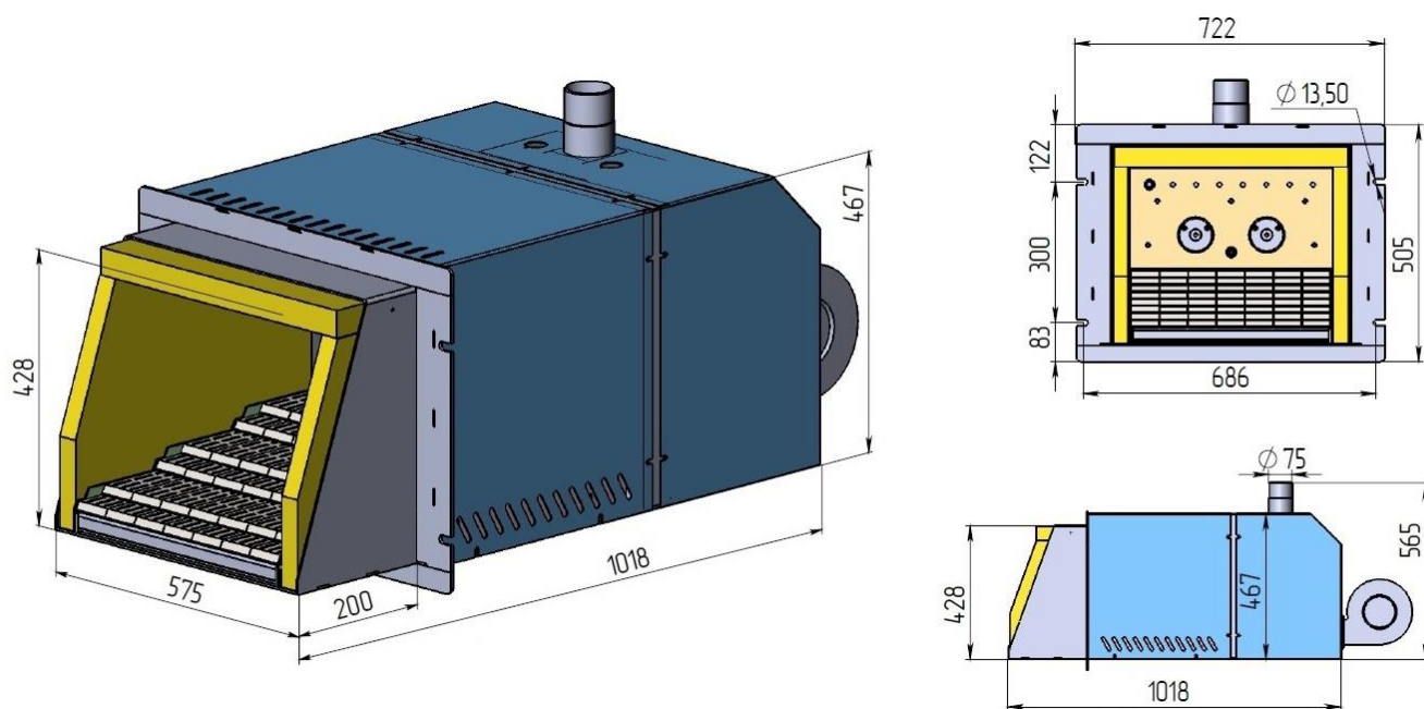
Мал. 1 - Габаритні розміри пальника «METALEX» 600 кВт
