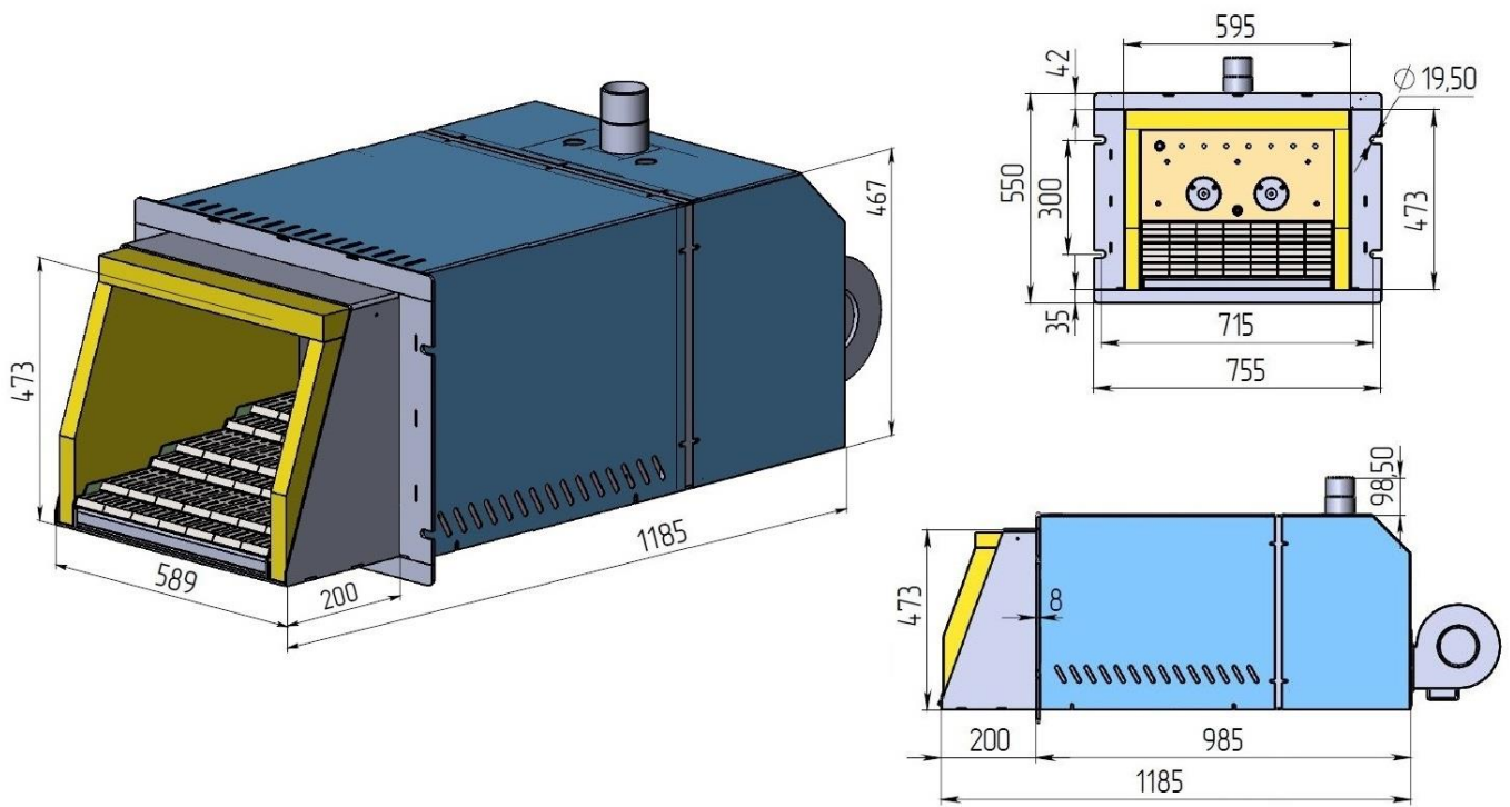
Мал. 3 - Габаритні розміри пального «METALEX» 800 кВт
