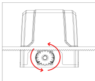
Обертаючись, вихідна шестерня приводить у рух раму воріт.
