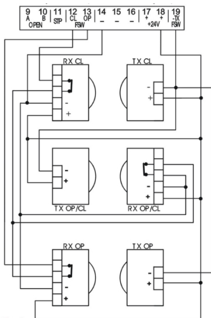
Подключение фотоэлементов на открывание сработка фотоэлементов приводит к открыванию
