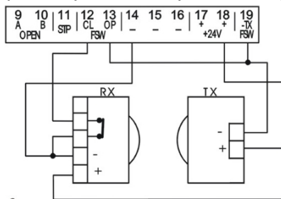
Подключение фотоэлементов на закрывание сработка фотоэлементов приводит к закрыванию
