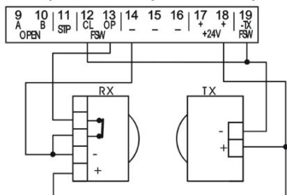
Подключение фотоэлементов на открывание сработка фотоэлементов приводит к открыванию
