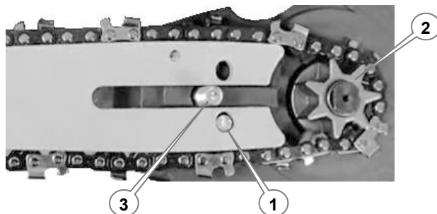
Рисунок 8. Схема встановлення різального блоку на виріб.
