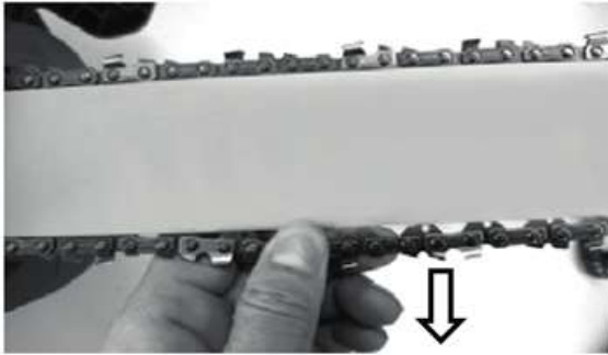
Рисунок 9. Схема перевірки натягу ланцюга.
