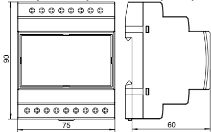
Рис. 1 Габаритные размеры
