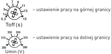
Rys. 2 Panel sterowania
