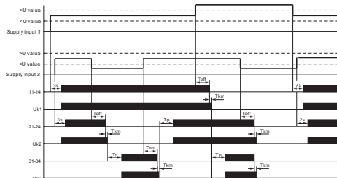
Рис. 3 Діаграма роботи
