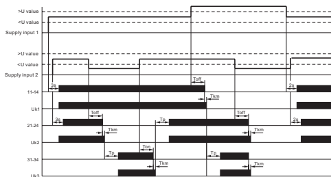
Рис. 3 Диаграмма работы
