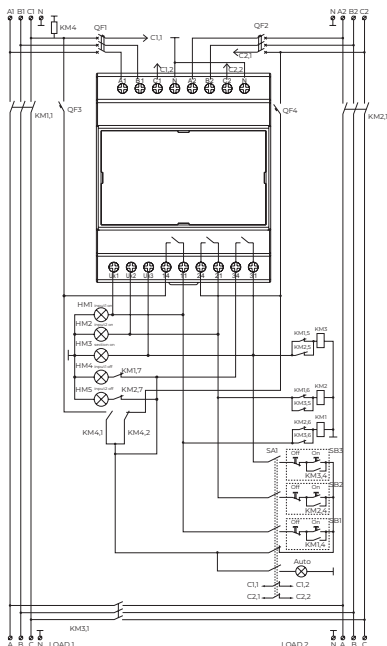
Rys. 4 Schemat połączenia ze stycznikami
