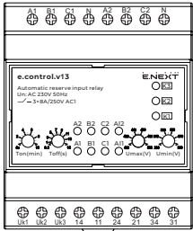
Des.2 Panou de control
