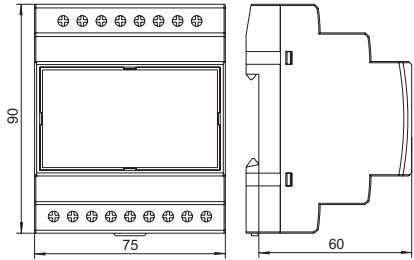
Rys. 1 Wymiary gabarytowe
