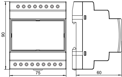
Рис. 1 Габаритни размери
