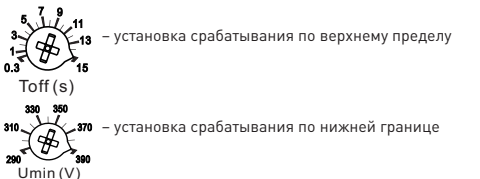
Рис. 2 Панель управления
