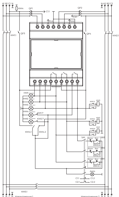
Рис. 4 Схема підключення з контакторами
