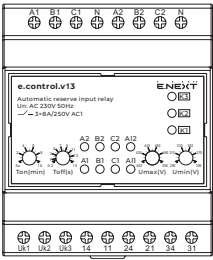
Rys. 2 Panel sterowania
