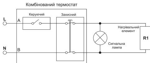
Рисунок 6. Схема електрична для моделей: D400S
