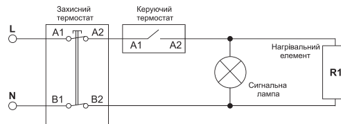
Рисунок 7. Схема електрична для моделей: D400S-1-BC, D400S-2-BC, D400S-2-B
