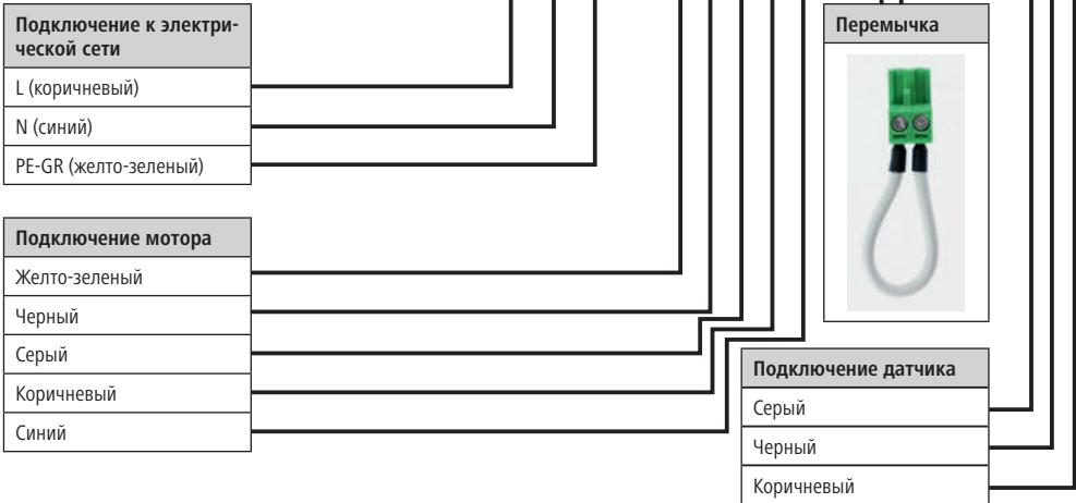
Рисунок 8. Схема подключения платы с конденсатором MaxiSwing
