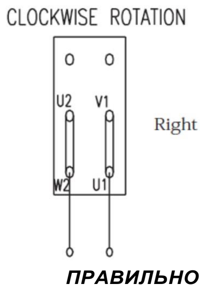
Рис. 14 – Схема електричних підключень насоса
