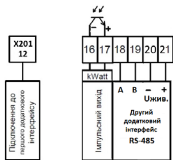
Рисунок 2 – Схема підключення інтерфейсів лічильника
