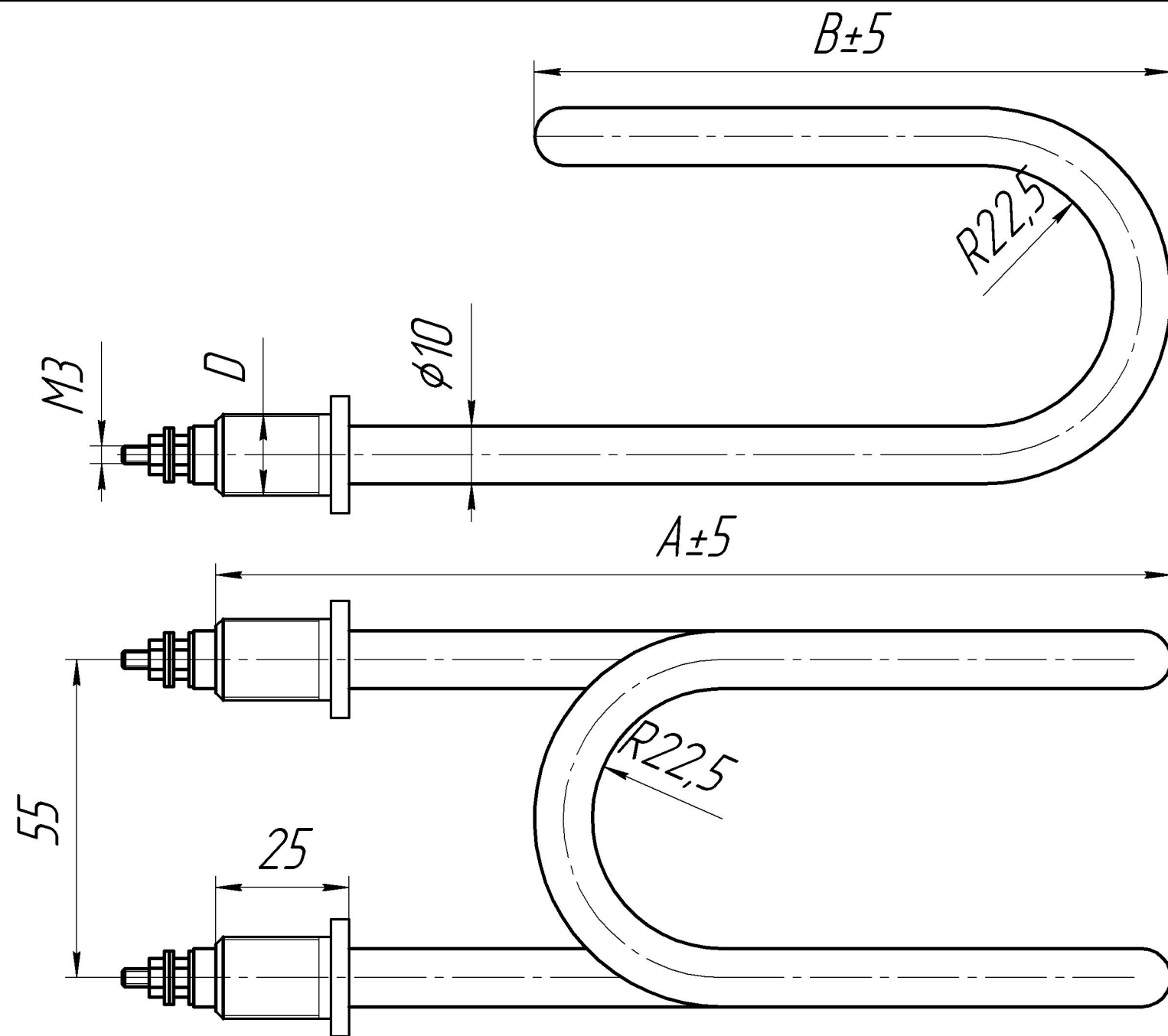
Трубчастий електронагрівач для дистиллятора медичного
