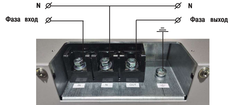
Рис.3. Схема подключения стабилизатора.
