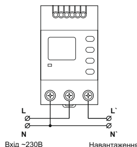
Схема підключення
