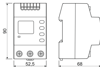
Габаритні розміри
