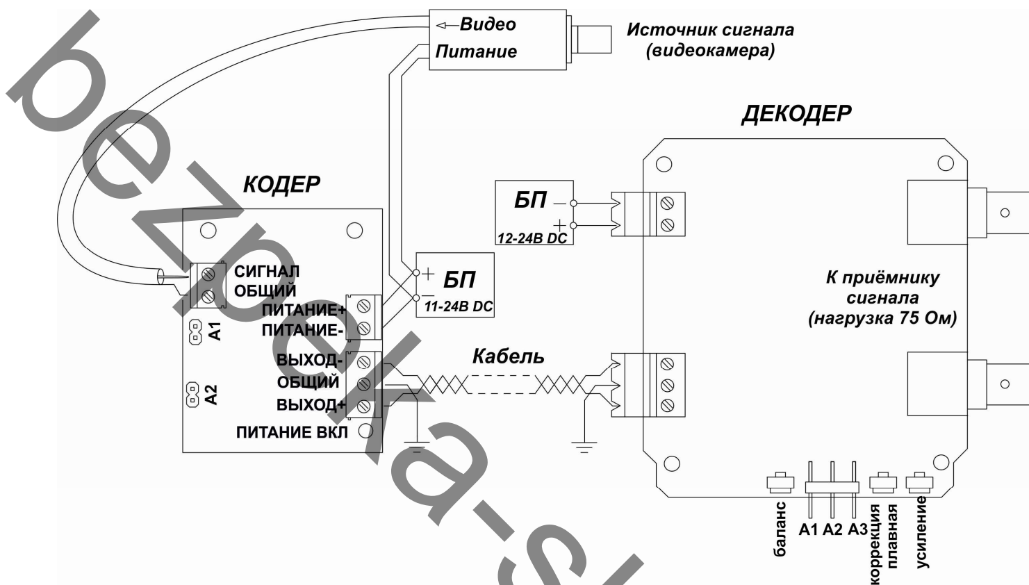
Рис. 1б Схема включения с двухсторонним заземлением (со стороны кодера и декодера).
