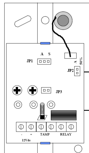
РИС. 2 – ПЕЧАТНАЯ ПЛАТА
