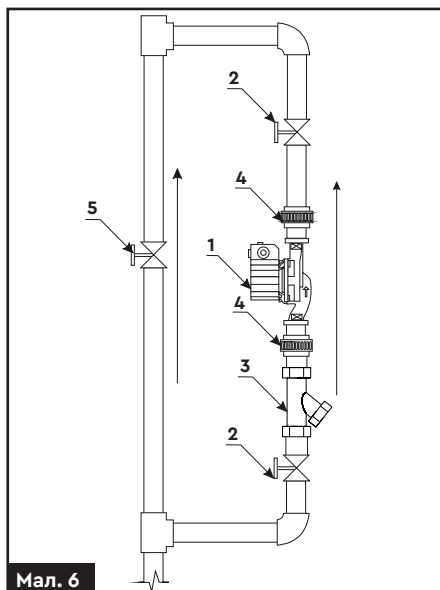
Мал. 6 – Схема монтажу насоса
