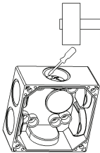
Рис. 3 Встановлення в отвори необхідних вставок-адаптерів під ізолюючу трубу або під герметичний ввід, відповідно: *
