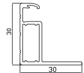
Переріз з довгої сторони рами
