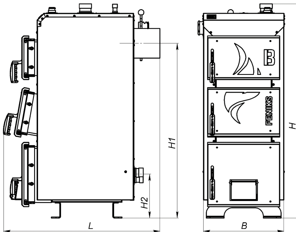
Рисунок 1 – Позначення габаритів котла
