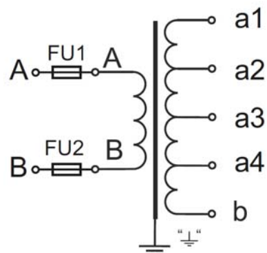
Рисунок А.2 – Схема электрическая принципиальная трансформаторов напряжения PVD1F-2.1.2-...//220-100-209-231
