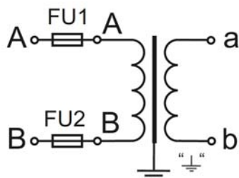
Рисунок А.1 – Схема электрическая принципиальная трансформаторов PVD1F-2.1.2-...//220
