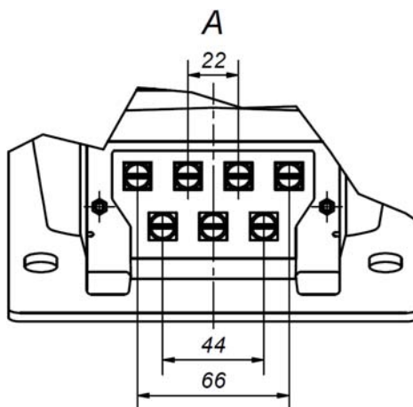
Рисунок Б.3 - Конструкция контактов вторичной обмотки трансформаторов напряжения
