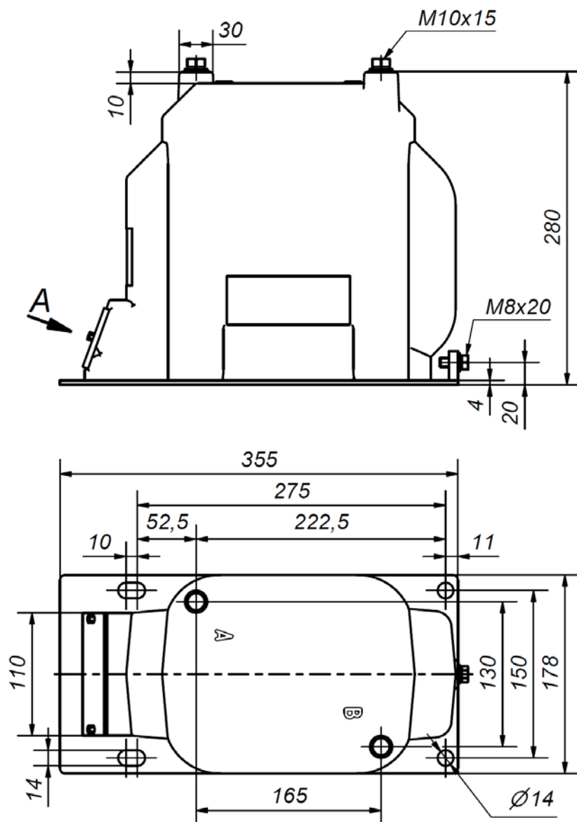
Рисунок Б.2 – Габаритный чертеж трансформаторов PVD1-2.1.2-...//220 и PVD1-2.1.2-...//100-209-220-231
