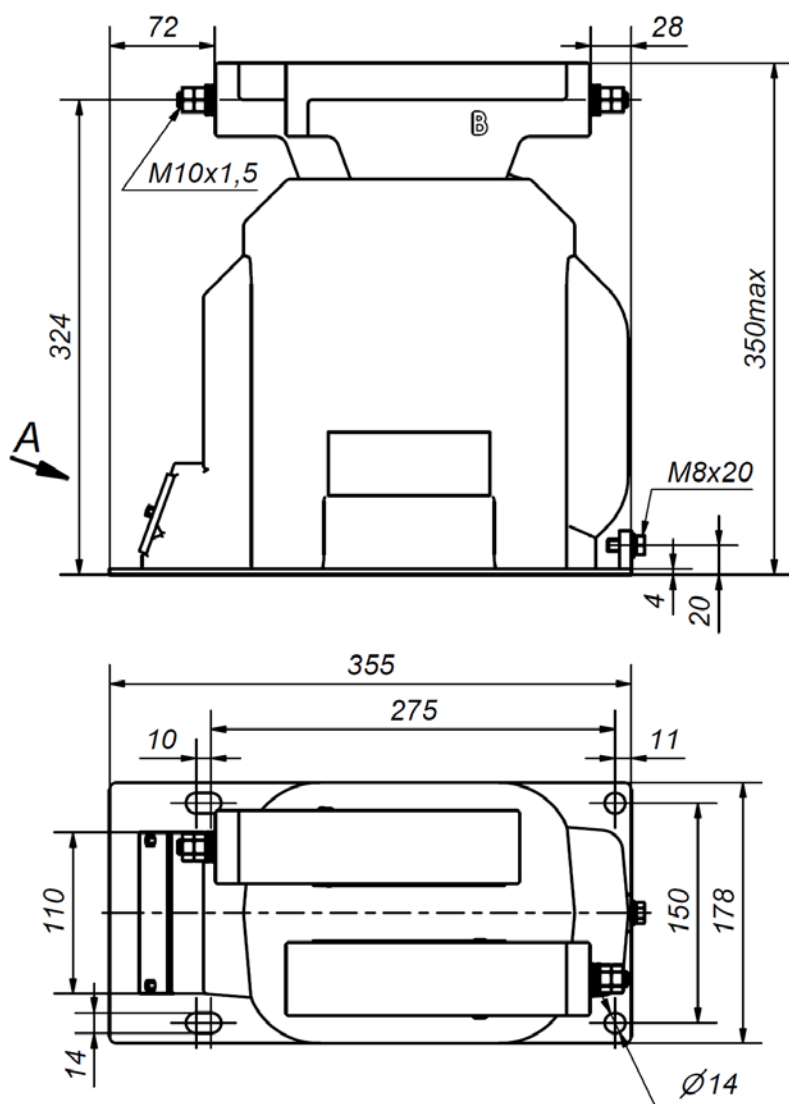
Рисунок Б.1 – Габаритный чертеж трансформаторов PVD1F-2.1.2-...//220 и PVD1F-2.1.2-...//100-209-220-231
