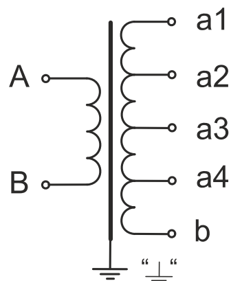
Рисунок А.4 – Схема электрическая принципиальная трансформаторов напряжения PVD1F-2.1.2-...//220-100-209-231
