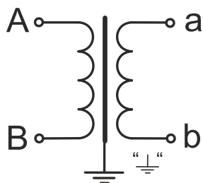
Рисунок А.3 – Схема электрическая принципиальная трансформаторов PVD1-2.1.2-...//220
