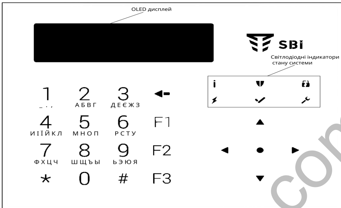
Рисунок 3 - Зовнішній вигляд клавіатури K-GLCD
