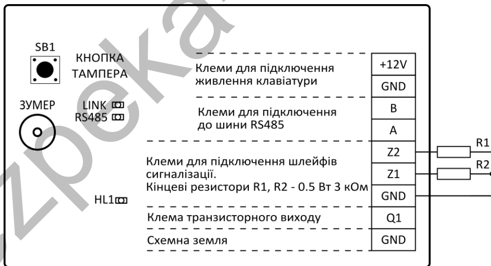
Рисунок 2 - Схема електрична підключення
