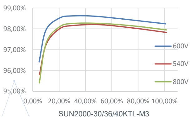
Крива ефективності
