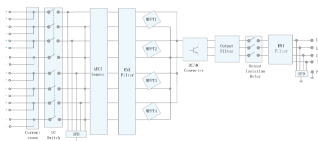
Принципова схема
