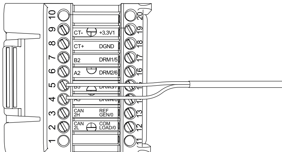
Малюнок 5-42 Схема з'єднання EMS
