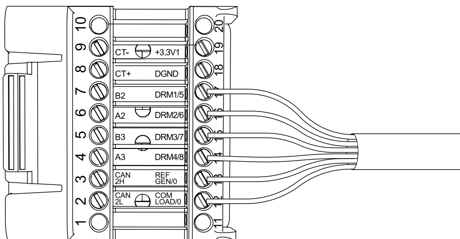
Малюнок 5-43 Схема з'єднання DRED
