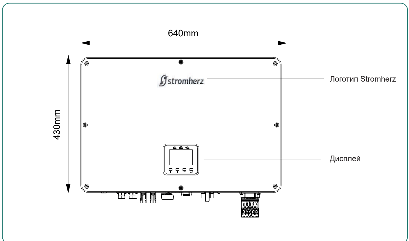
Малюнок 3-3 Вигляд спереду
