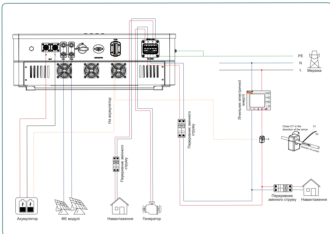
Малюнок 5-1 Стандартна схема електропроводки
