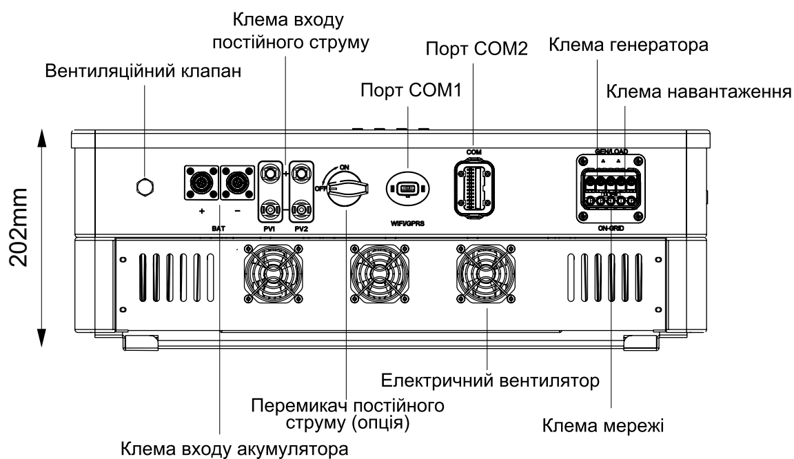
Малюнок 3-5 Вигляд знизу
