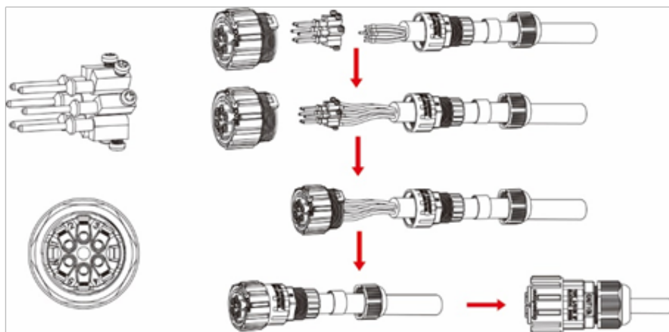
Малюнок 4.24 Роз'єм DRM
