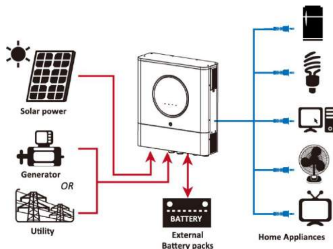
Малюнок 1 Базовий огляд гібридної PV-системи
