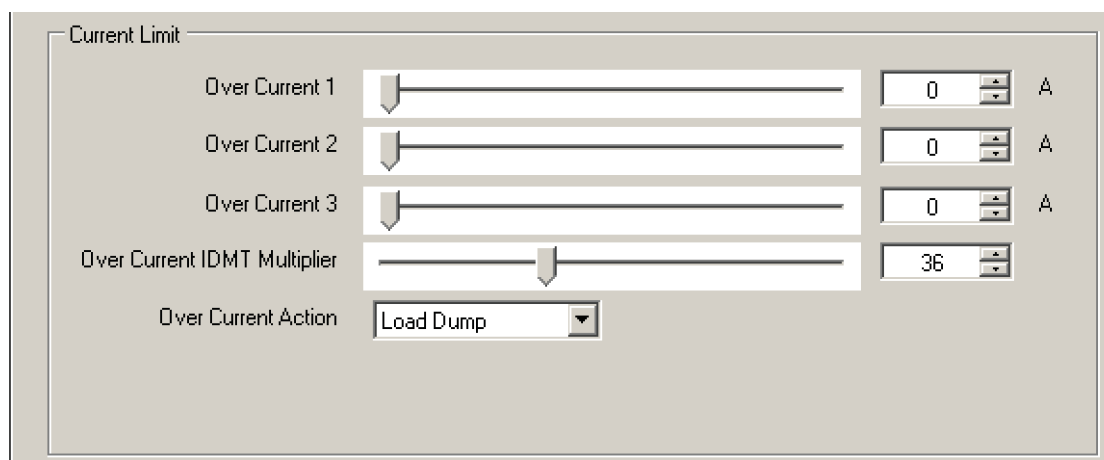
Знімок екрана з програми налаштувань RainbowPlus, розділ Generator>Current (Генератор>Ток)
