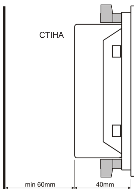
Необхідна глибина стійки керування
