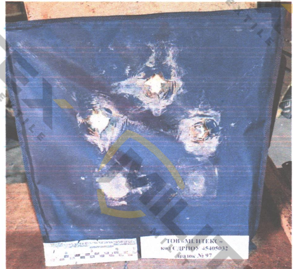
Фото 1.1.1. Зразок № 97 до та після випробування (за нормальних умов).
