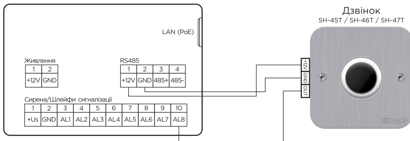
Схема підключення кнопки як дверного дзвінка
