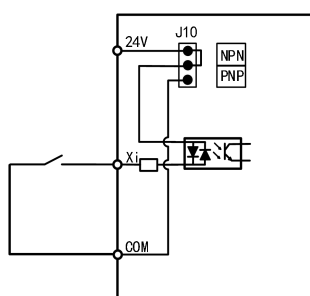
а: Со встроенным питанием в NPN режимет
