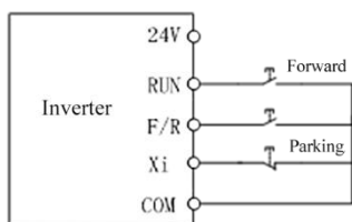
(a) Трехпроводное управление (F00.03=2)
