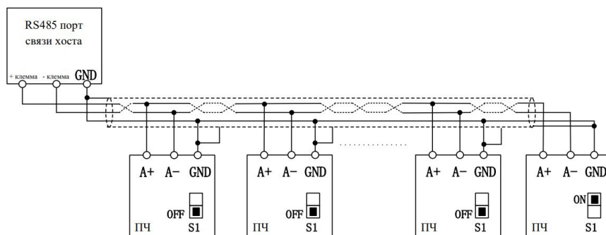
Рис. 3-17 множественное подключение частотных преобразователей
