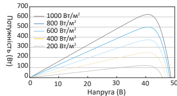
Крива «потужність-напруга» JAM66D45-625/LB
