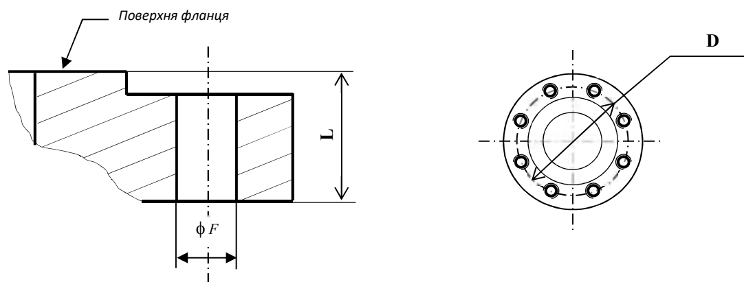
Рисунок 12. Параметри фланцевих з'єднань лічильників Delta™ S3F з номінальними діаметрами 150 мм.
