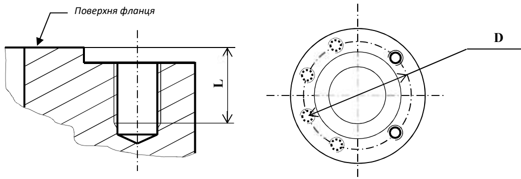
Рисунок 11. Параметри фланцевих з'єднань лічильників з номінальними діаметрами до 100 мм включно.
