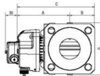
Фланцева версія — DELTA Compact DN25 / DN40 / DN50
