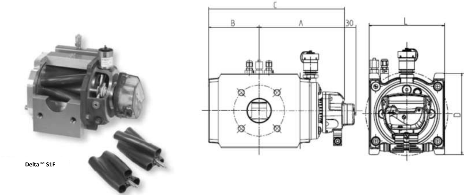
Рисунок 10. Зовнішній вигляд і габаритні розміри лічильників Delta™ S1F
