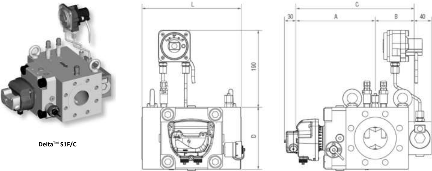
Рисунок 9. Зовнішній вигляд і габаритні розміри лічильників Delta™ S1F/C
