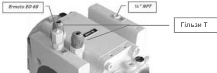
Рисуюнок 3. Розташування штуцерів і гільз на корпусі лічильника
