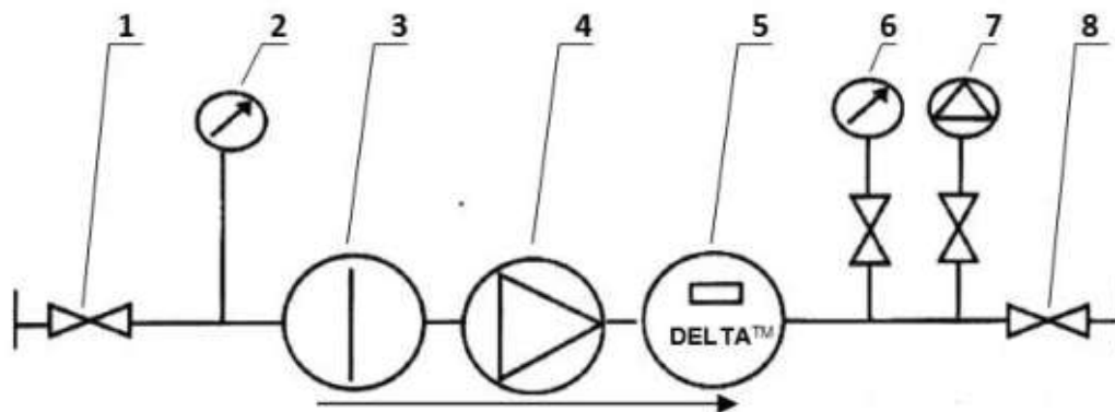
1, 8 — запірні вентилі, 2, 6 — манометри, 3 — основний фільтр, 4 — регулятор тиску газу, 5 — лічильник DELTA™, 7 — запобіжно-спускний клапан.
