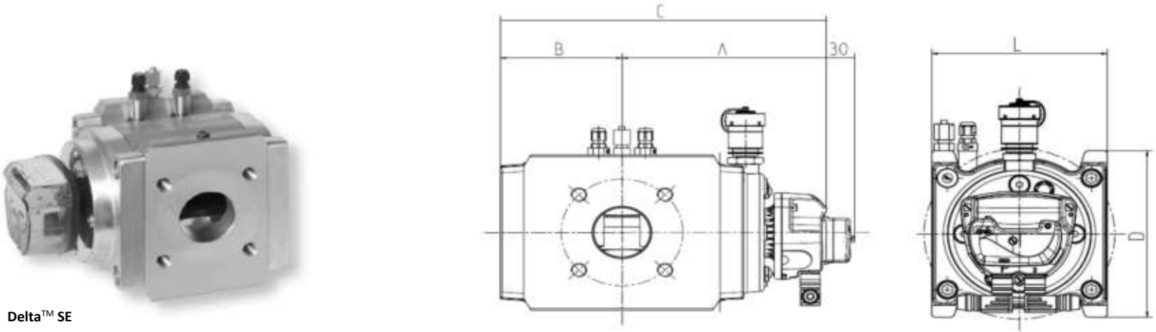
Рисунок 6. Зовнішній вигляд і габаритні розміри лічильників Delta™ SE
