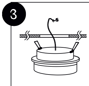
3. Зафіксувати ліхтар у стелі за допомогою пружин
