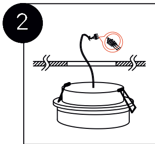
2. З'єднати кабель живлення лампи з мережним кабелем живлення
